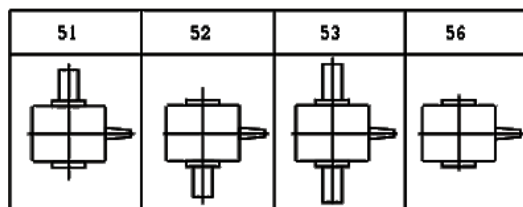
Варианты сборки редукторов
