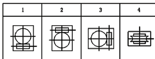
Варианты расположения червячной пары в редукторах
